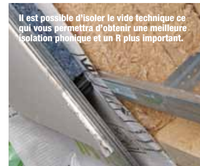
d) Suspente + fourrure + membrane + Sixbox® ou tasseau de bois (vide technique 15 mm à 100 mm) + fourrure
