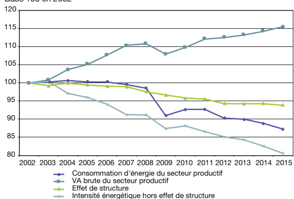
Graphique 6 : décomposition de l'évolution de la consommation d'énergie du secteur productif en France
