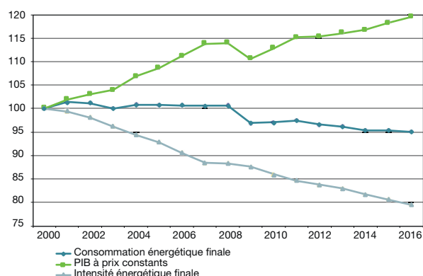
Graphique 1 : décomposition de l'évolution de la consommation énergétique finale de la France
