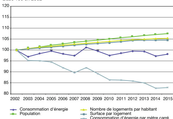
Graphique 3 : décomposition de l'évolution de la consommation d'énergie résidentielle en France
