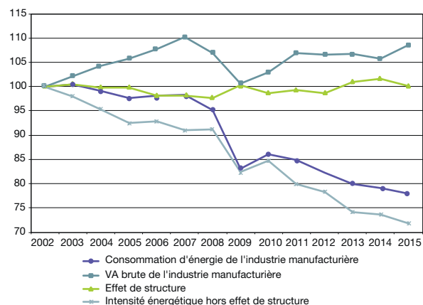
Graphique 7 : décomposition de l'évolution de la consommation d'énergie de l'industrie manufacturière en France Base 100 en 2002
