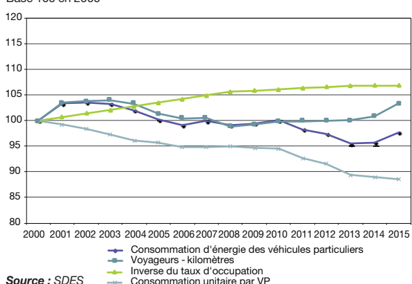
Graphique 4 : décomposition de l'évolution de la consommation d'énergie des véhicules particuliers en France
