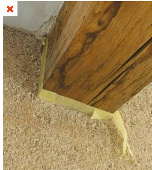
Noircissement d'une poutre apparente suite au contact avec la chaux. ©AQC-2015
