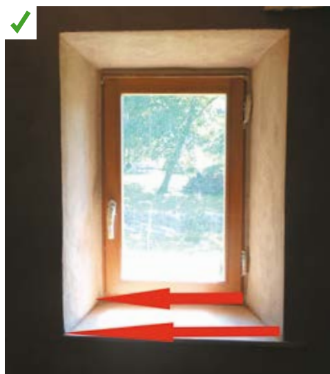
Travail d'ébrasement incliné lors d'une rénovation thermique intérieure. ©AQC-2015
