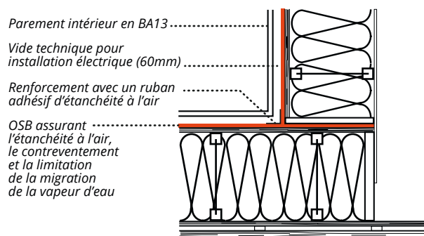
Jonctions entre panneaux OSB jointoyées avec un adhésif adapté. ©AQC-2015
