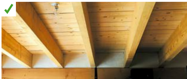
Protection du bois avec l'huile de lin avant la projection. ©AQC-2015
