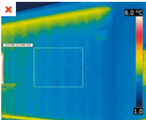
Thermographie d'une paroi isolée en ouate de cellulose. ©AQC-2015
