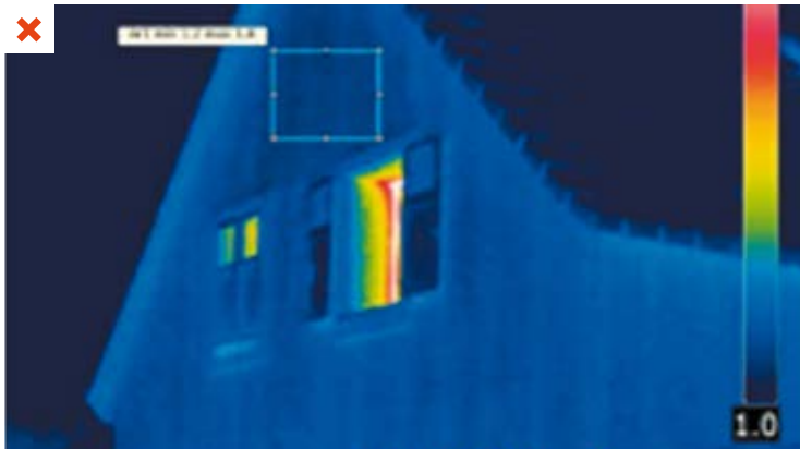
Thermographie d'une paroi montrant la faiblesse thermique des montants en bois de l'ossature porteuse avec isolation en bottes de paille. ©AQC-2015
