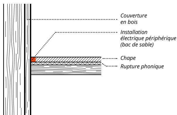
Intégration des installations électriques à la périphérie d'un plancher bois. ©AQC-2015
