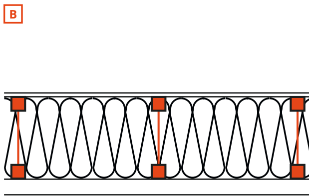
Montants en « I » pour diminuer les ponts thermiques. ©AQC-2015
