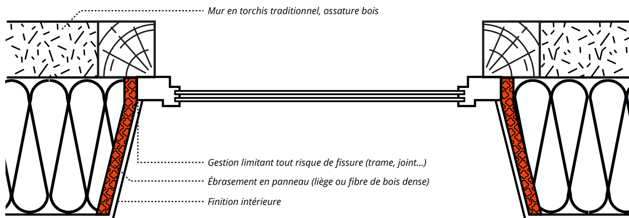
Détail d'ébrasement en panneau de liège ou fibre de bois. © AQC-2015
