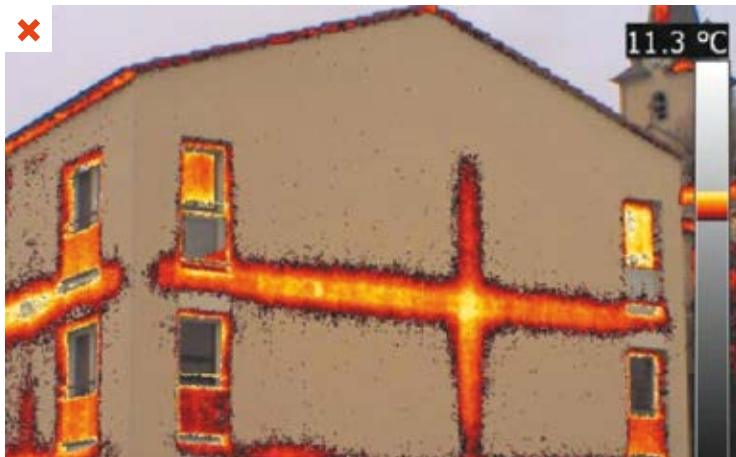
Photo thermique des déperditions au niveau des planchers et murs en rénovation thermique intérieure. ©FLIR Systems
